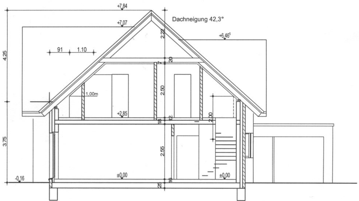
Schnitt A-A
